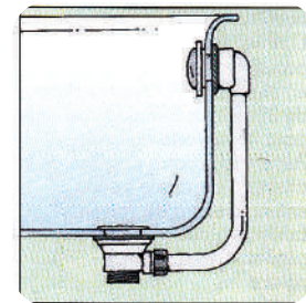
Desagüe para bañera
