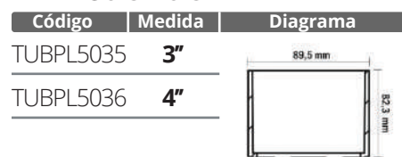
Adaptador para tubo redondo
