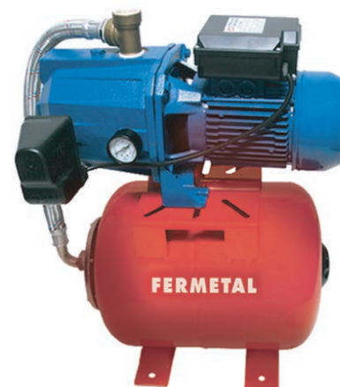
Bomba hidrocompacto de 1 HP
